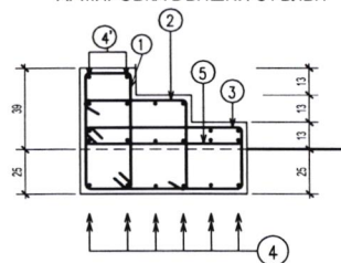
АРМИРОВКА ВЪНШНИ СЪЛБИ
