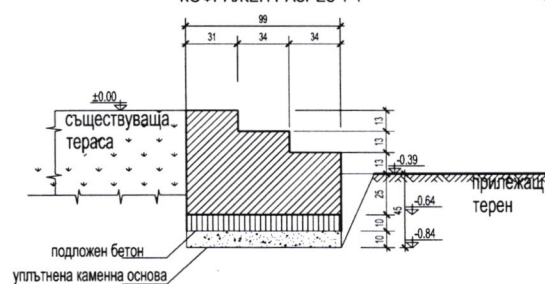
КОФРАЖЕН РАЗРЕЗ 1-1
