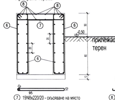
Армиране тераса
