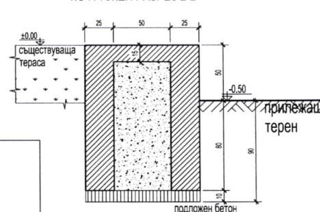
Армиране тераса
