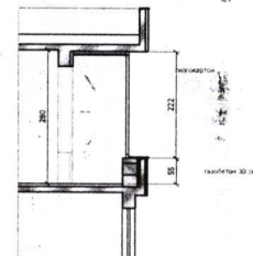
РАЗРЕЗ 3-3
