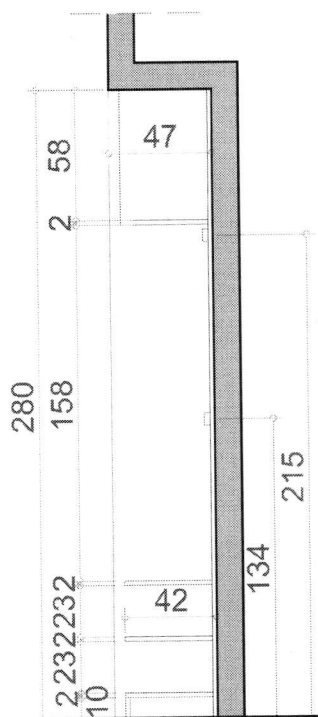
Вертикален разрез 1-1
