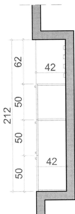
План
