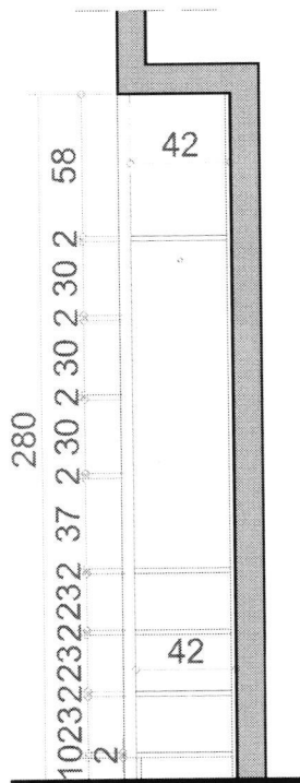
Вертикален разрез 2-2
