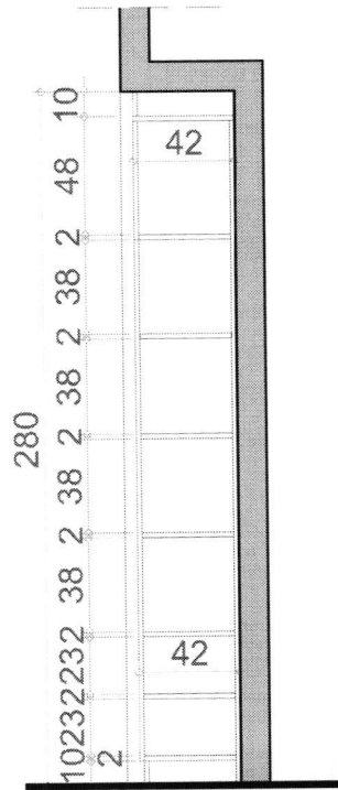
Вертикален разрез 3-3
